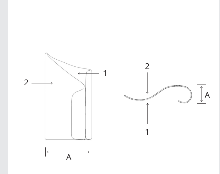
Seitenansicht / Draufsicht side view / top view
